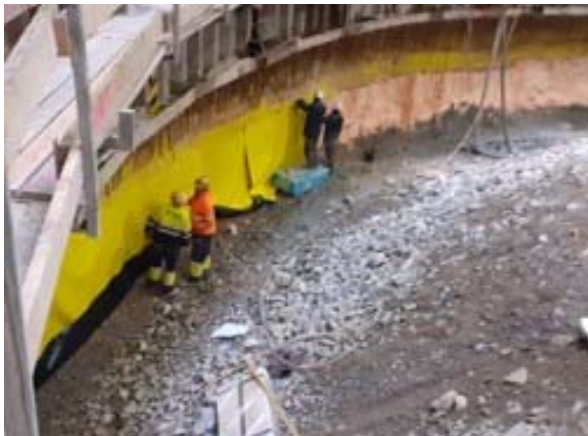
Impermeabilització de l'anell 11
